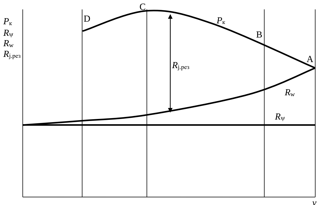
Рисунок 10 - График тягового баланса автомобиля
