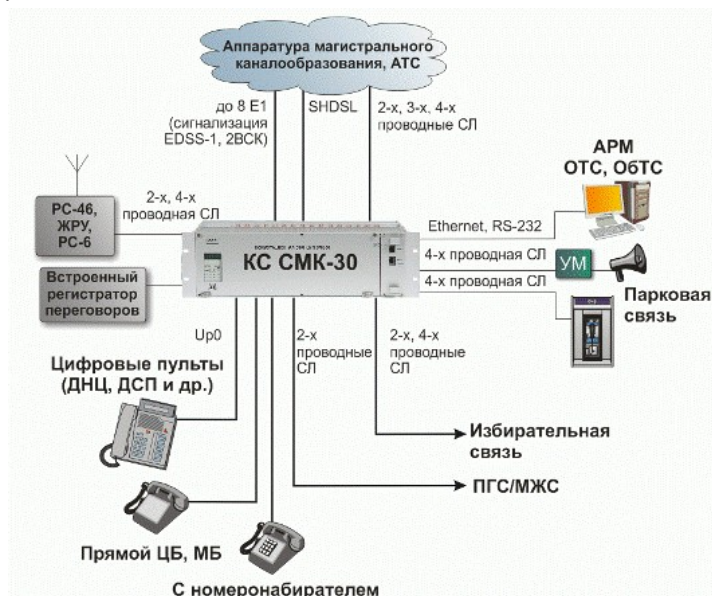
Рисунок 1.1 - Структурная схема аппаратно-программного комплекса связи на SMK-30
