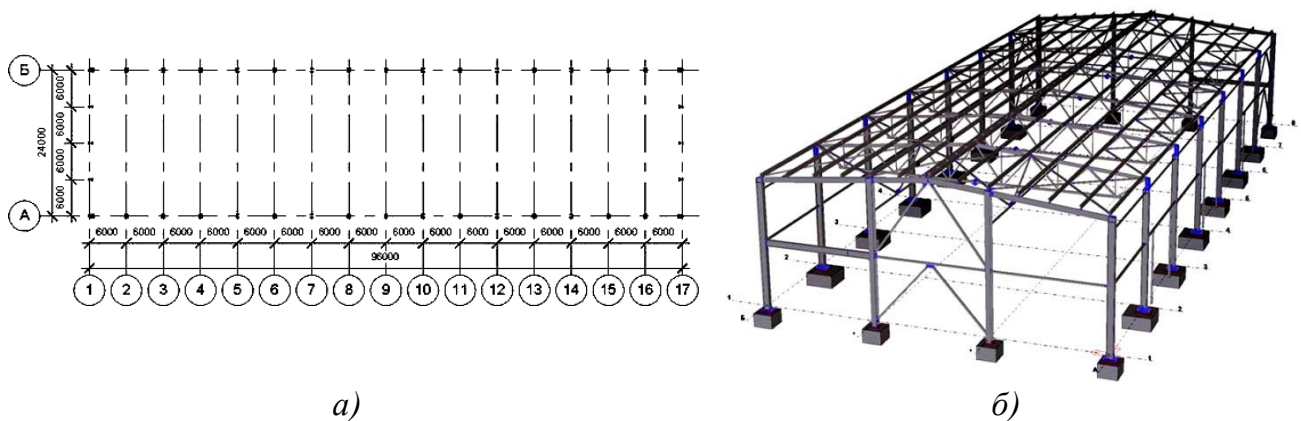
Рисунок 6.1 – Компонка здания производственного корпуса АТП а) конструктивная схема; б) 3D модель
