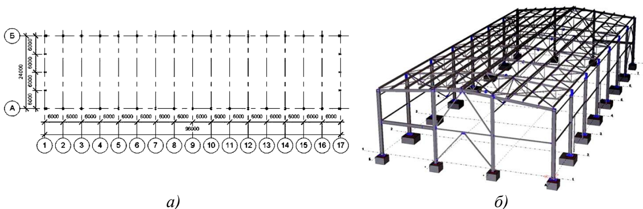
Рисунок 6.1 – Компонировка здания производственного корпуса АТП
