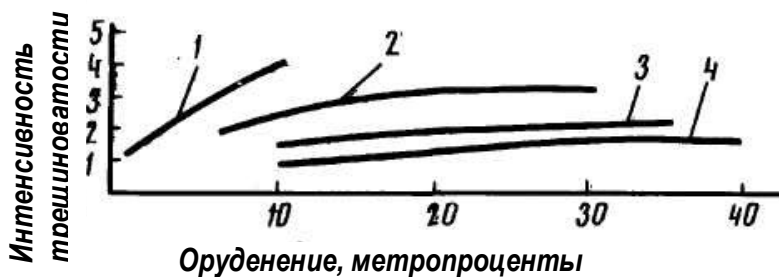
Рис. 3.16. Зависимость интенсивности трещиноватости ( W ) от оруденения ( C ): 1 – залежь «Покро 7а»; 2 – залежь «Кресто – 9»; 3 – залежь «Покро – 7»; 4 – залежь «Покро – 8».
